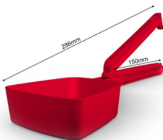
WELOC SCOOP PA 150-250, PA 220-250 Y PA 320-250
