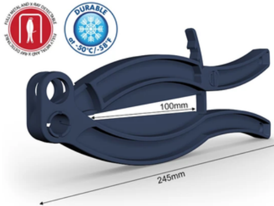
WELOC DETECTABLE GRIPPER POM 100 FD ●
