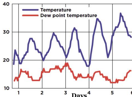
Transporte con control del punto de rocío La temperatura del punto de rocío se mantiene por debajo de la temperatura superficial, lo que evita la condensación y los daños por humedad and moisture damage.
