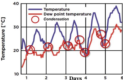
Transporte sin control del punto de rocío La condensación se produce cuando la temperatura superficial y la temperatura del punto de rocío son iguales.
